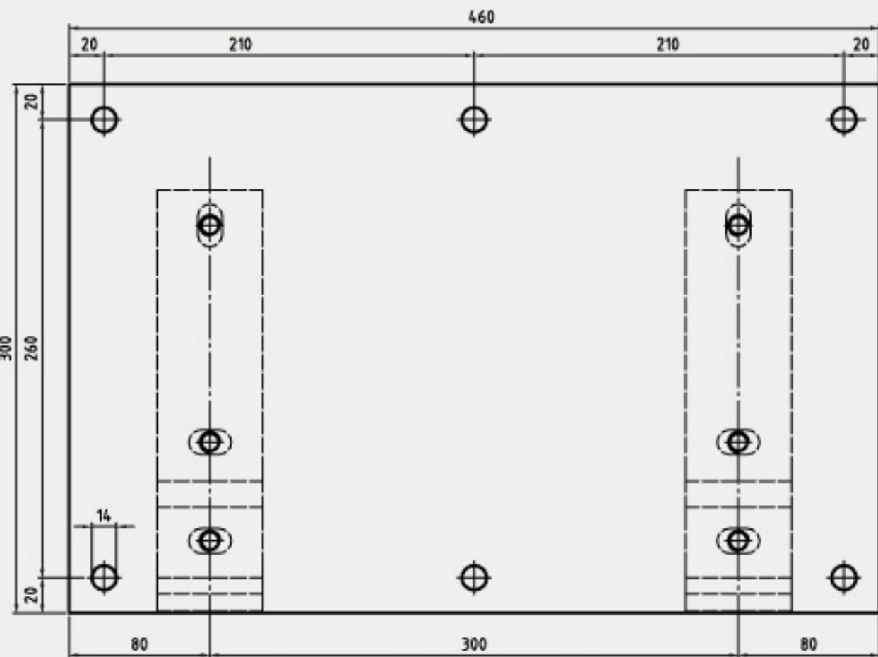
Montageplatte MP300 / 2x60er Wand
