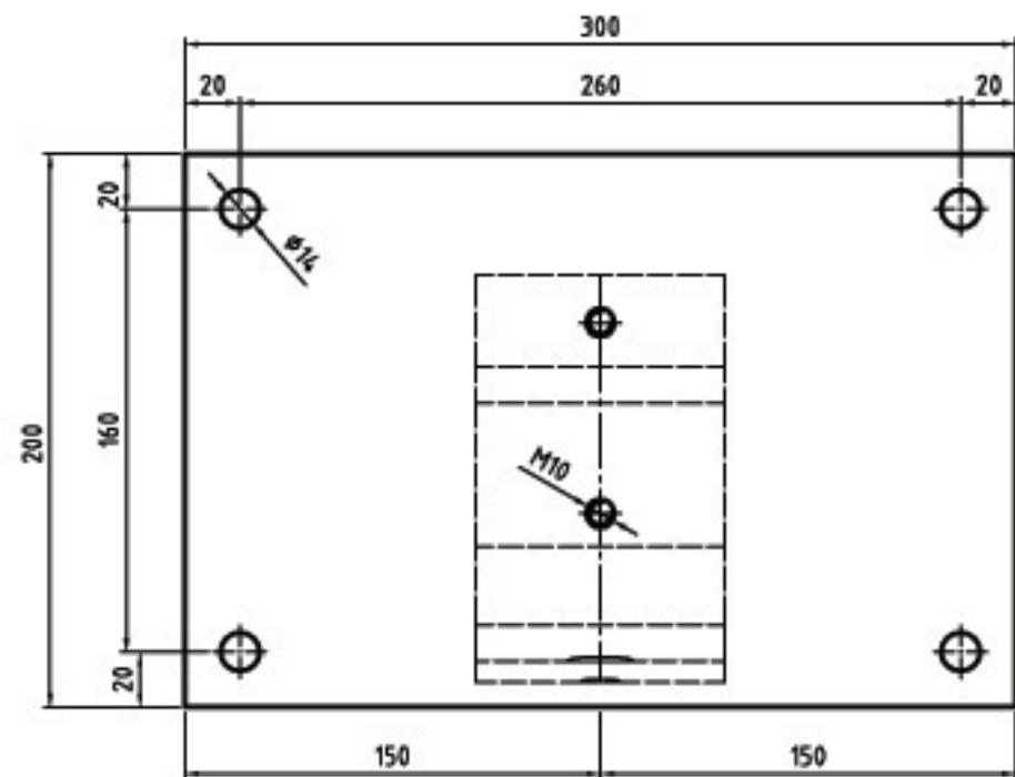
K400 Montageplatte MP200-1x90er Deckenmontage
