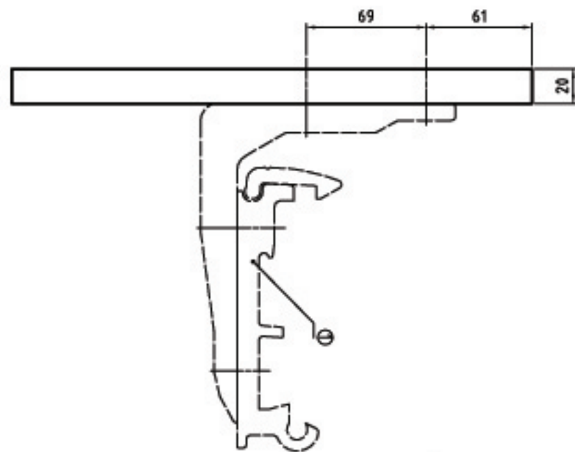
K400 Montageplatte MP300-1x90er Deckenmontage
